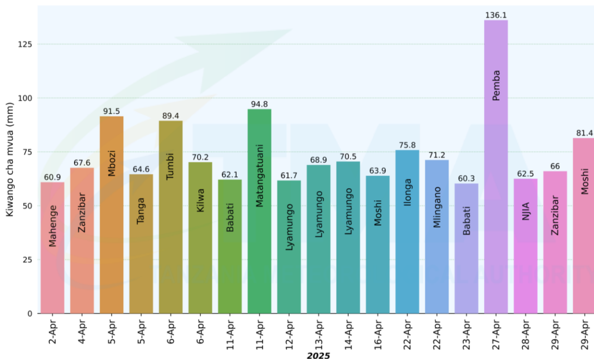
Kielelezo 1: Vituo vilivyopima viwango vya mvua milimita 60 au zaidi katika mwezi Aprili, 2025
